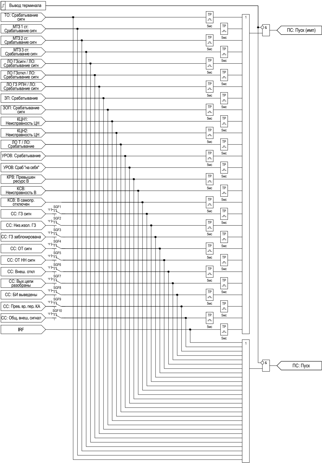
Рисунок 2.31 – Функциональная схема «ПС»
