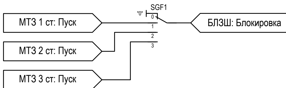
Рисунок 2.4 – Функциональная схема БЛЗШ
