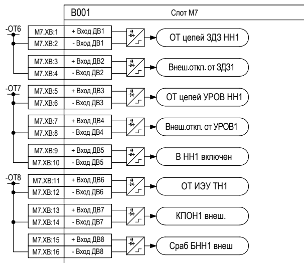
Рисунок Ж.3 – Подключение дискретных входов и выходов к внутренним сигналам алгоритмов для плат в слотах М6-М8
