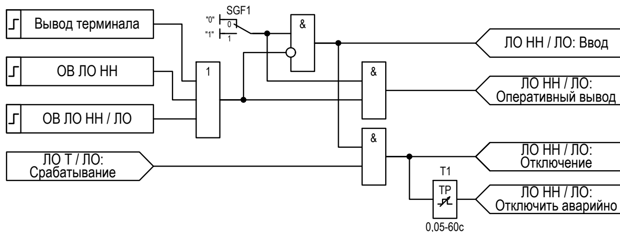
Рисунок 2.19 – Функциональная схема «ЛО»
