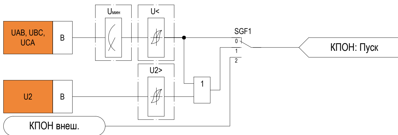
Рисунок 2.2 – Функциональная схема «КПОН»
