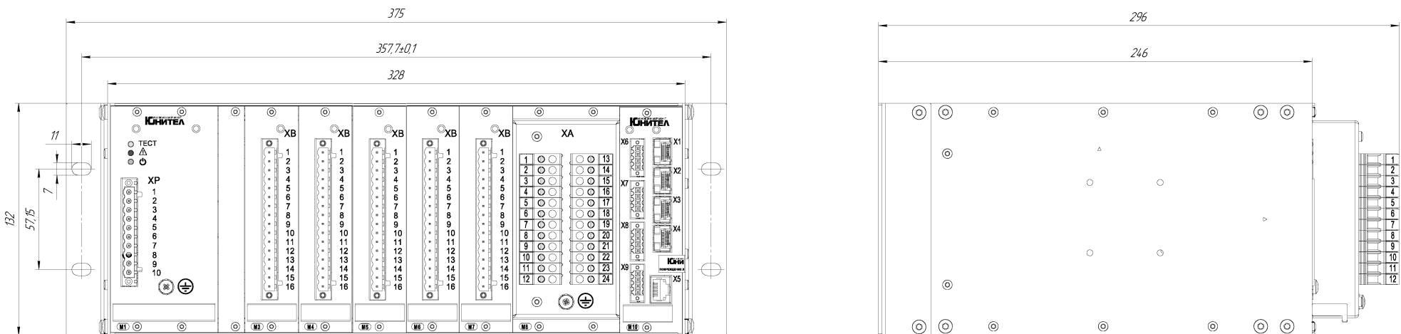
Рисунок Г.2 – Габаритные и установочные размеры устройства в исполнении ЮИТЕ-М314-Т2 (II архитектура)
