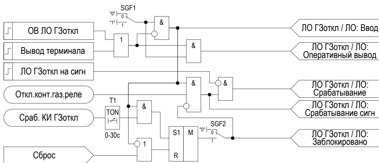
Рисунок 2.12 – Функциональная схема «ЛО ГЗоткл»
